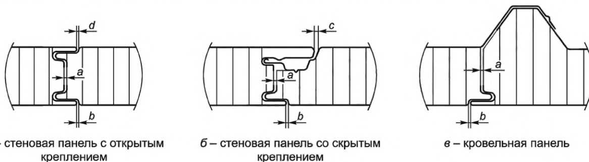
Рисунок 25 — Схема измерения зазора по сердечнику в монтажном положении и отклонения от номинального значения зазора облицовок в монтажном положении
